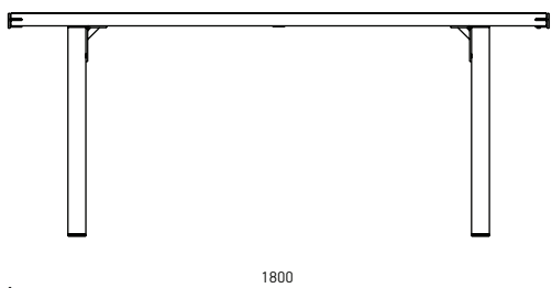
Klaar Steel table - KLST180
