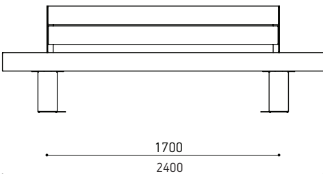
Nippon-penkki 2400 mm selkänojalla - NIPB240-04
