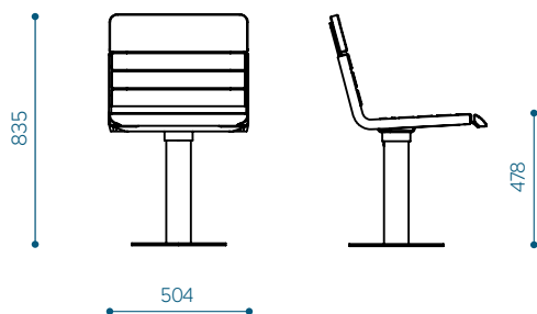
Hula tuoli, ilman käsinojia - HUB50
