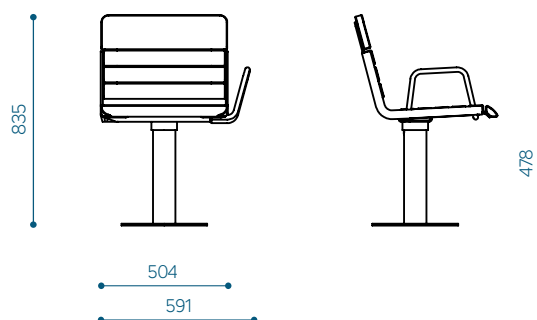
Hula tuoli, vasemmalla käsinojalla - HUB50-05
