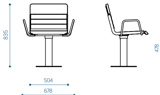
Hula tuoli, 2:lla käsinojalla - HUB50-02
