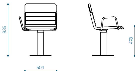
Hula tuoli, oikealla käsinojalla - HUB50-04
